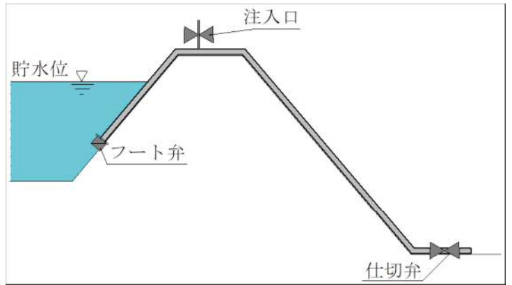
図1 整備する放流機能の仕組み
